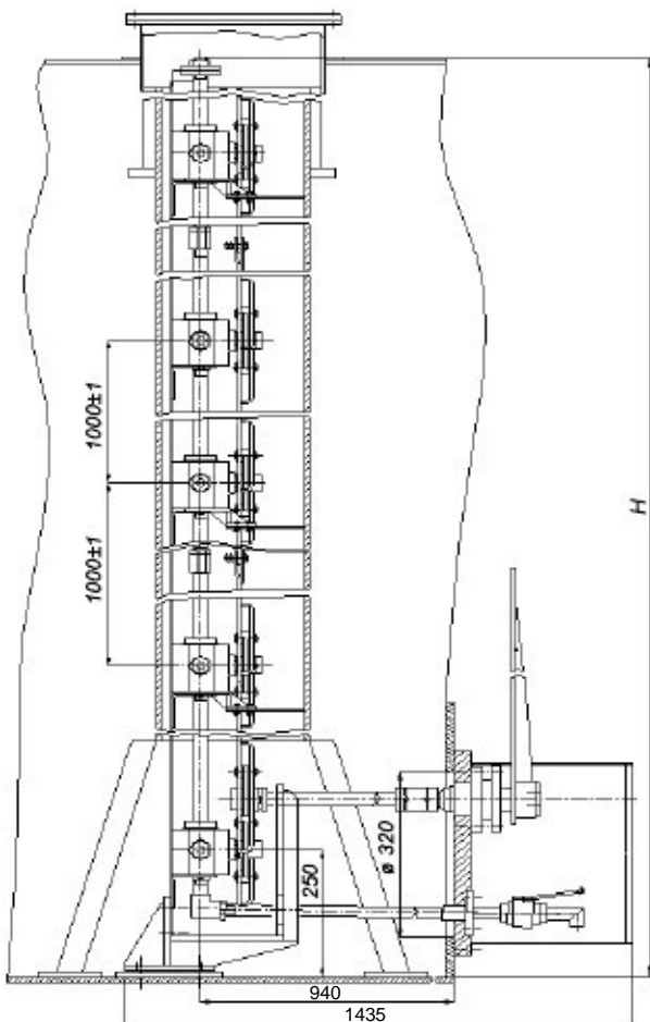
Общий вид пробоотборника секционного ПСРП
